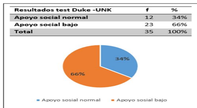
Gráfico 1. Resultados de la aplicación del test Duke-UNC
